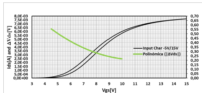
Fig. 6. Curva característica de ingreso IDS-VGS (linear-linear) del dispositivo A @ -5V a 15V.
