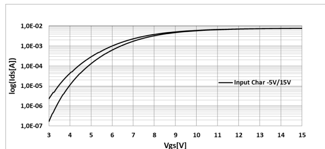
Fig. 7. Curva característica de ingreso IDS-VGS (logarítmica-linear) del dispositivo A @ -5V a 15V.
