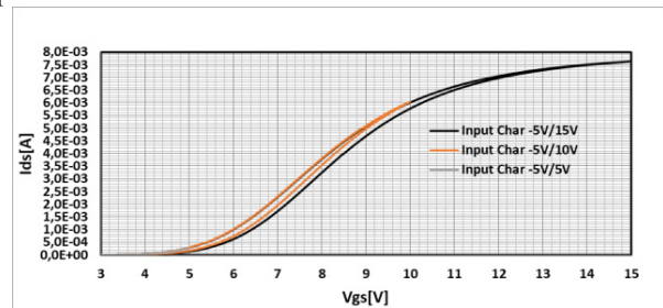
Fig. 5. Comparación entre las curvas características ingreso IDS-VGS (linear-linear) (dispositivo A).
